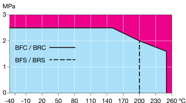
Grafik 1. Druck-Temperatur-Diagramm.
