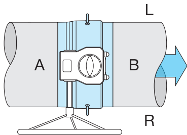
Abbildung 26. Installationsposition AR.
