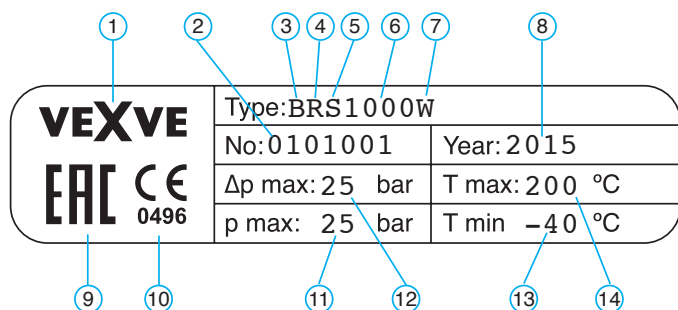
Abbildung 1. Typenschild.
