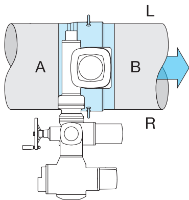
Abbildung 30. Installationsposition ARA.
