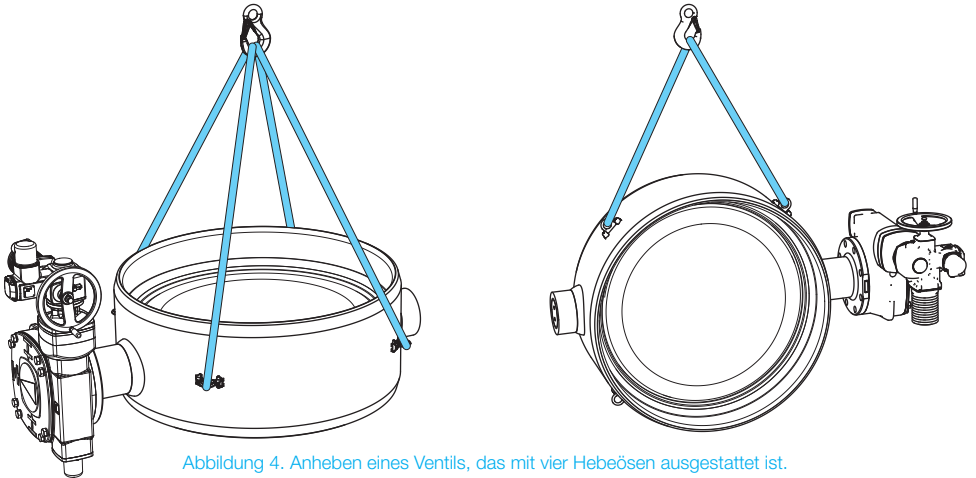
Abbildung 4. Anheben eines Ventils, das mit vier Hebeösen ausgestattet ist.
