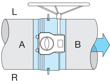
Abbildung 27. Installationsposition AL.
