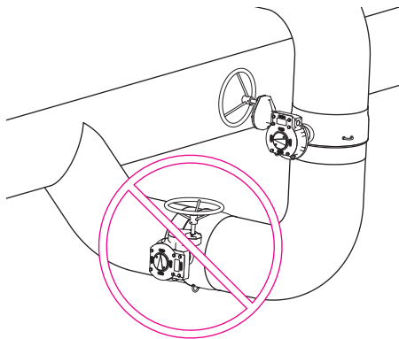
Abbildung 10. Ventilplatz.
