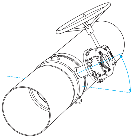
Abbildung 13. Installation in einem Winkel.
