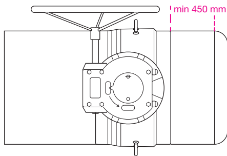
Abbildung 17. Blindflansch.
