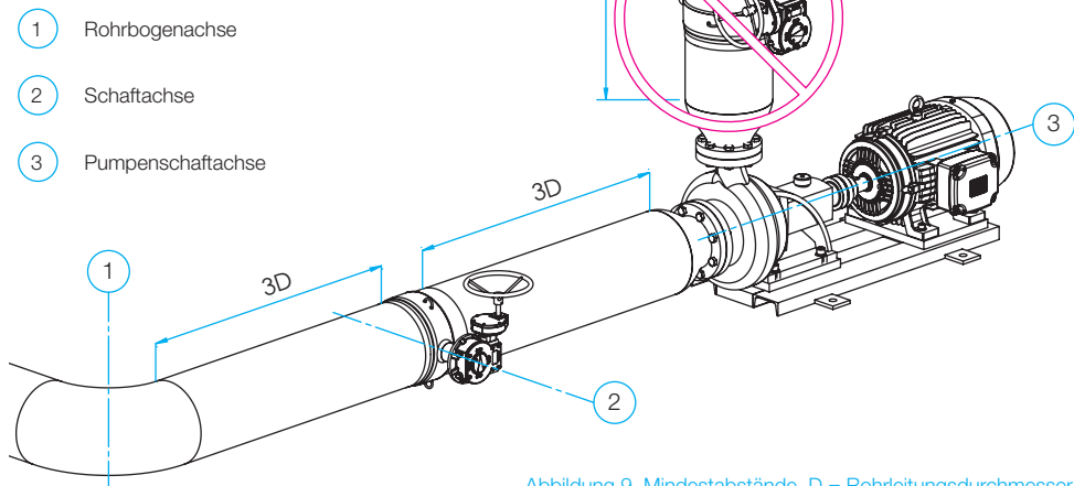
Abbildung 9. Mindestabstände, D = Rohrlungsdurchmesser.
